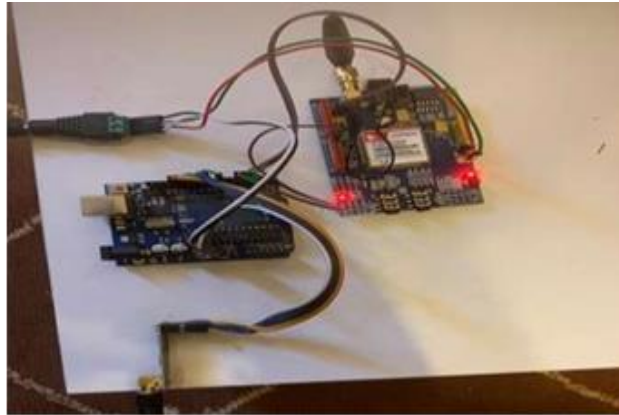
Fig 3 Slave unit.
